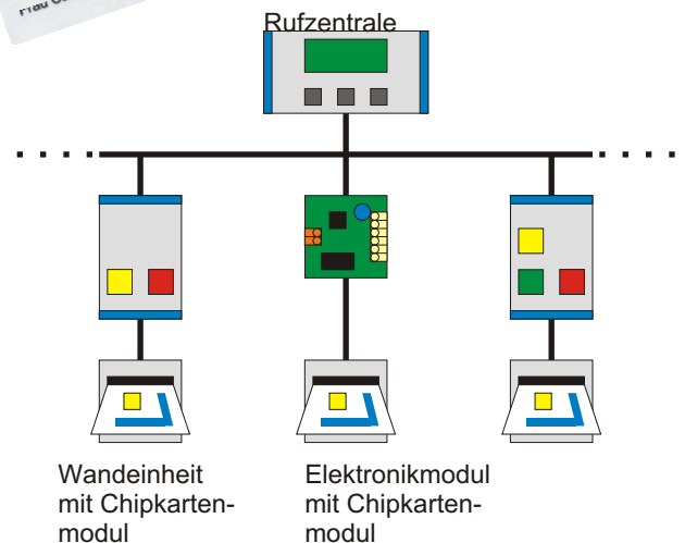
Abbildung: Rufsystem gutCALL 4DB mit Chipkartenmodulen in den Zimmern
